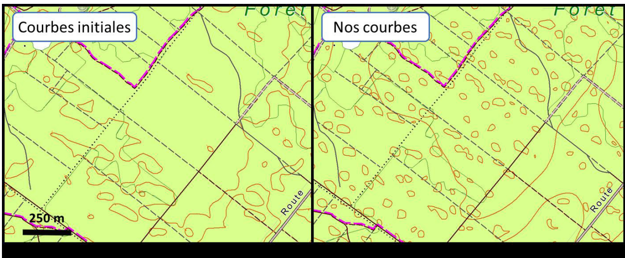
Figure 16 : Courbes de niveau obtenues avec la méthode présentée, intégrées dans la carte topographique au 1: 25k et comparées à la carte actuelle.
