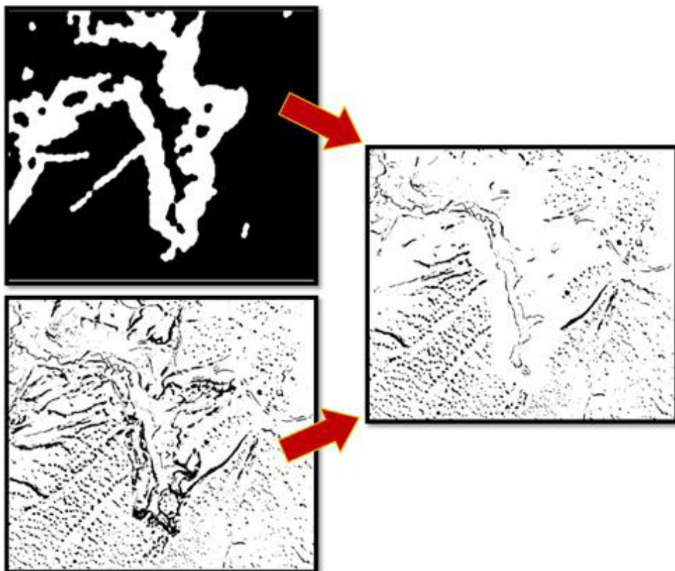
Figure 6 : Illustration des étapes (2.1) à (2.3) avec le masque plat / en pente en haut à gauche, la différence entre les MNT donnant des dépressions d'une profondeur supérieure à 1,5 mètre et, à droite, les dépressions situées dans une zone plate.
