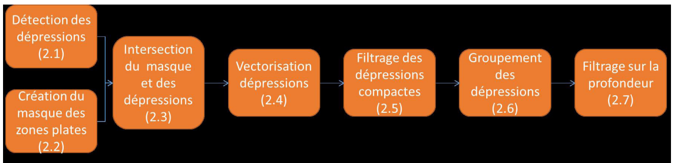
Figure 5 : Le processus de l'étape (2) avec les sept sous-étapes de la détection des dolines.
