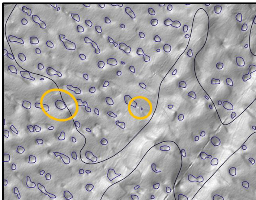
Figure 15 : Courbes de niveau finales affichées en haut du MNT. Les courbes en noir sont celles du cMNT et les courbes en bleu sont celles qui ont été ajoutées avec exagération des dolines. Les zones entourées montrent les problèmes restants.
