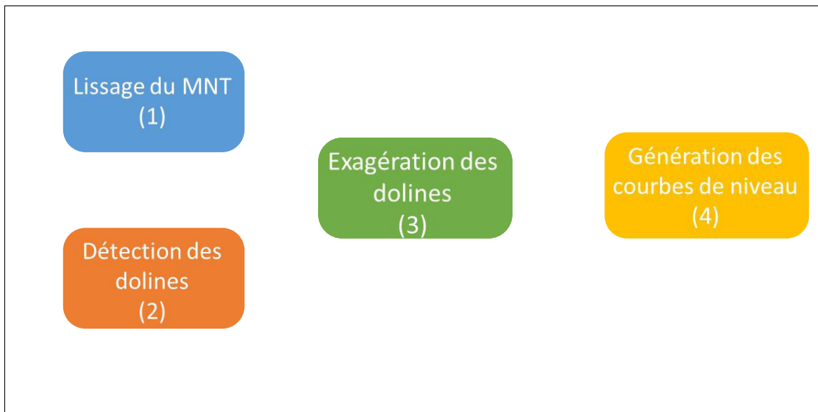
Figure 3 : Les quatre étapes principales du flux de travail pour obtenir des courbes de niveau de haute qualité sur les plateaux karstiques.
