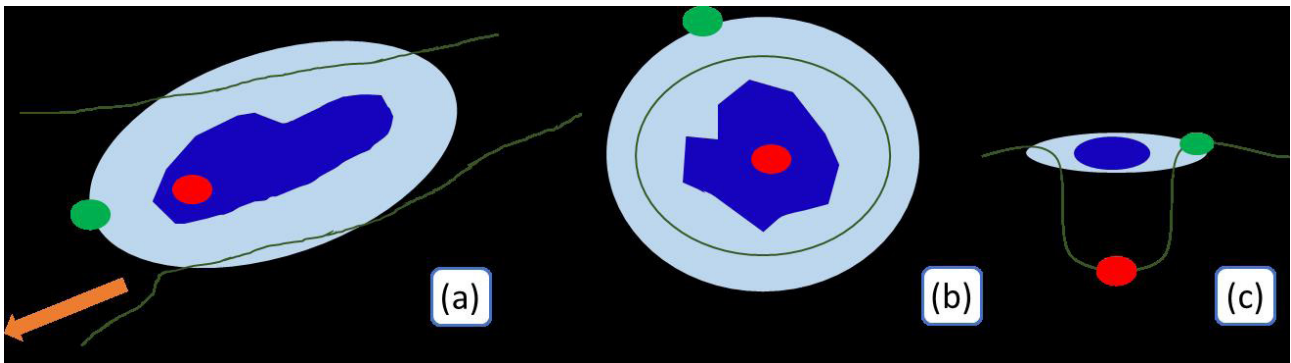
Figure 9 : Le point vert représente l'altitude minimale du contour de la zone dilatée, le point rouge représente l'altitude minimale de la doline détectée (a) un thalweg ; (b) une doline; (c) vue en coupe de la doline.
