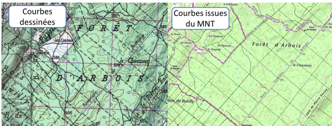
Figure 2 : Courbes de niveau dessinées manuellement sur l'image de gauche, générées à partir du MNT sur l'image de droite, dans un plateau rempli de dolines.
