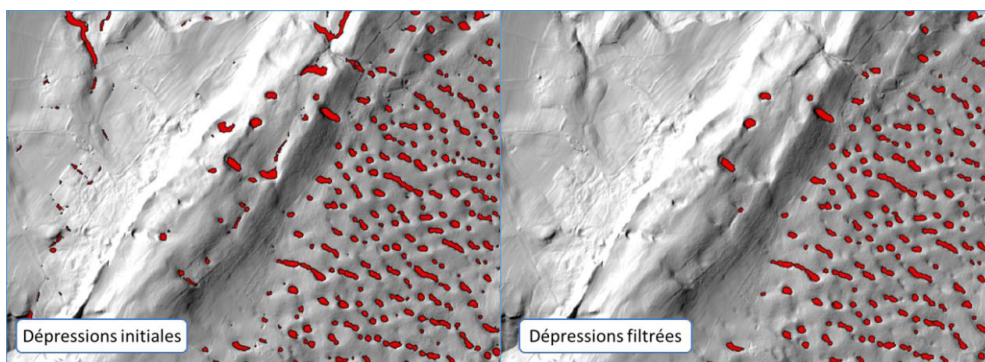
Figure 14 : Dépressions au-dessus du MNT avant et après l'étape de filtrage.
