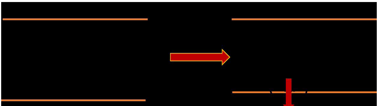
Figure 10 : Quand une doline a des altitudes maximales et minimales entre deux altitudes de courbes successives, l'altitude de la doline est ajustée pour intersecter l'altitude de la courbe de niveau la plus proche.
