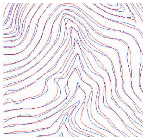
b) Courbes de niveau issues du nouveau MNT recalculé avec les lignes de cassure (rouge) et les courbes de référence(bleu)
