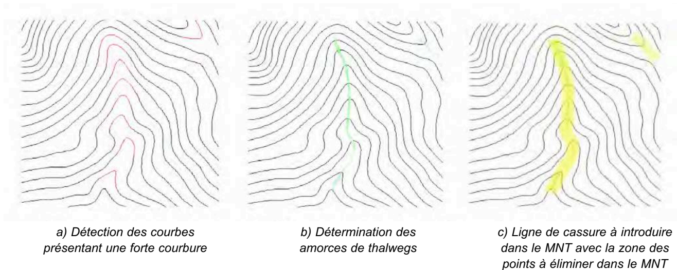
Figure 7: Processus de création des lignes de cassure à introduire dans le MNT
