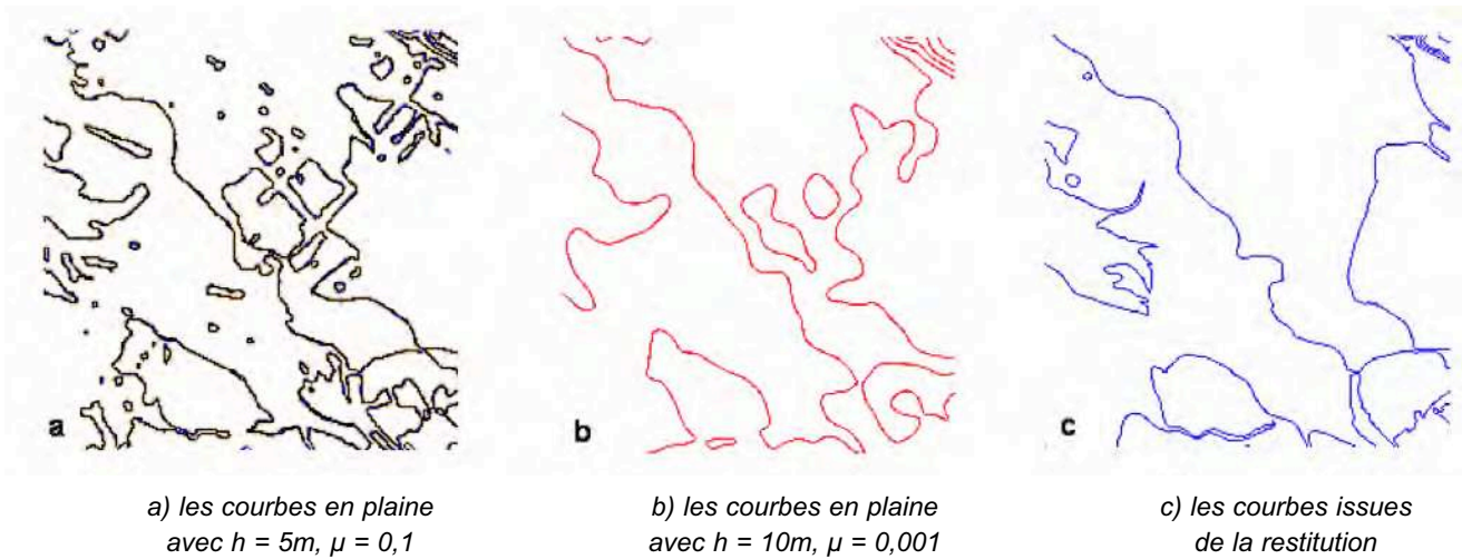
Figure 6 : Choix des paramètres de la grille élastique en plaine pour obtenir un rendu similaire à celui obtenu par un restituteur
