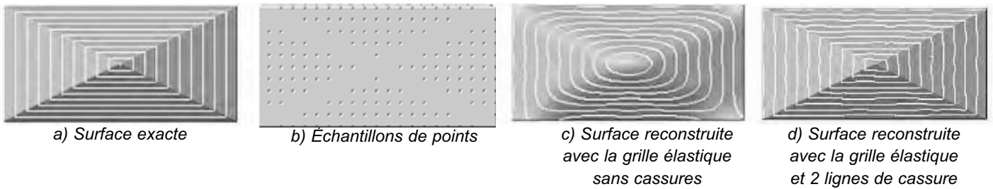
Figure 5 : Effet de l'introduction de lignes de cassure dans la grille élastique pour la reconstruction de surface à partir d'un échantillon de points
