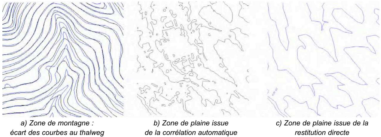
Figure 4 : Comparaison des courbes obtenues par restitution (en bleu, servant de référence) et les courbes calculées à partir du MNT à pas de 1m issu de la corrélation automatique (en noir)
