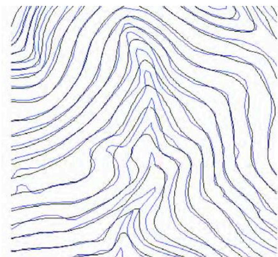
a) Courbes de niveau issues du MNT brut (noir) et les courbes de référence issues de la restitution (bleu)
